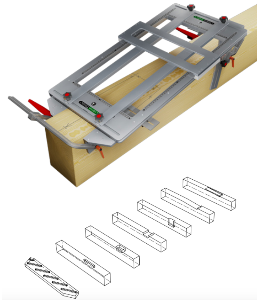
Nastavení úhlu pomocí stupnice s procenty a stupni
